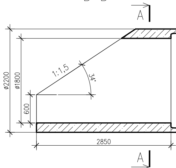
PRZEKRÓJ B-B
